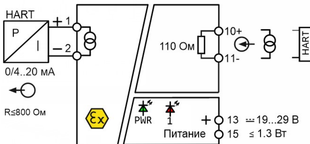
Рисунок 4.2.1 – схема подключения модуля I18Ex-AO-11-DC
