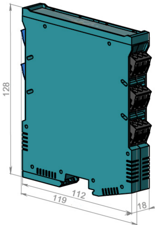
Рисунок 2.1 – габаритные размеры модулей (для справок)
